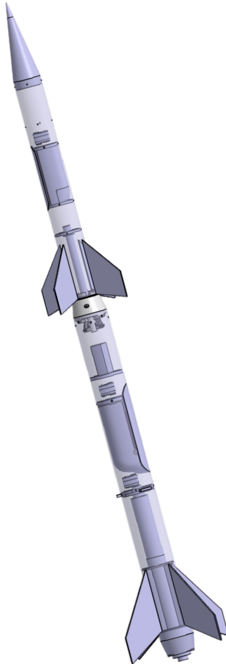
FIGURE 1.4 – Vue d'ensemble de la fusée SP-02 sur Openrocket
